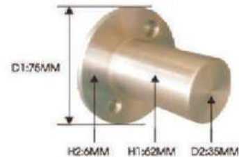
FLANGE SHAFT D1 75 mm D2 35 mm H2 6mm
